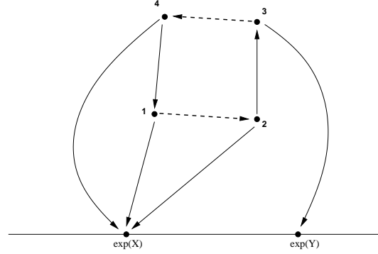
Roue pure taille 4 sur X, X, X, Y (3.7)
