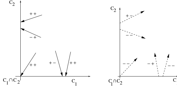
FIG. 2 – Fonction d'angle à 4 couleurs
