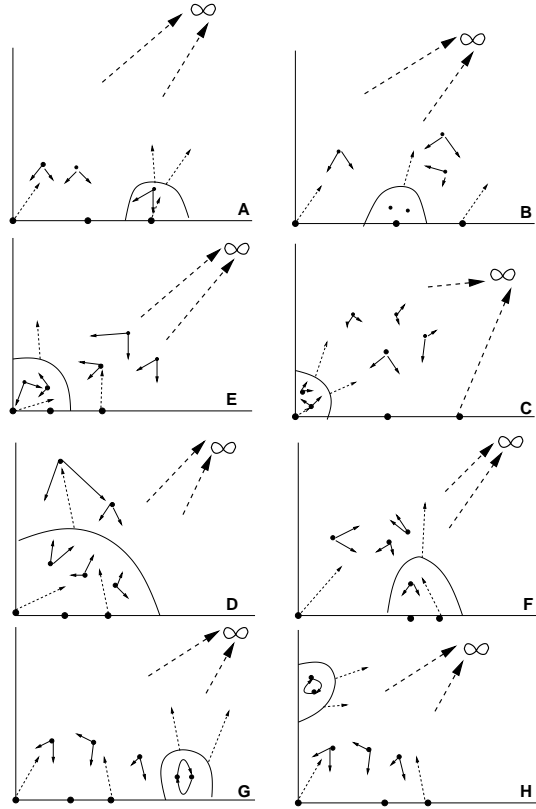
FIG. 3 – Diverses strates pour la compatibilité de l'action à droite en cohomologie
